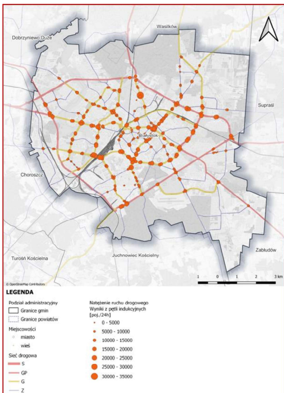
Rysunek 3.9 Obciążenie ruchem sieci drogowej Białegostoku Źródło: opracowanie własne na podstawie danych ZDM Białegostok
